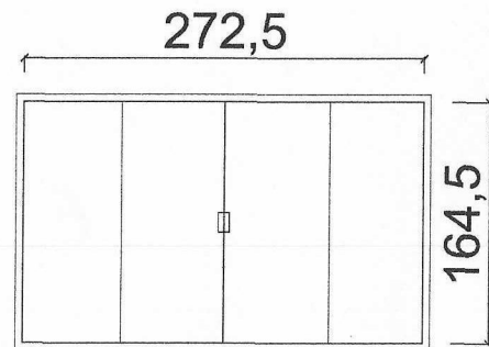
Janela Vidro Temperado 8mm incolor
