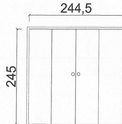
Porta Vidro Temperado 10mm incolor
