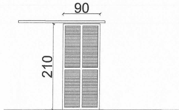
Porta de Correr Alumínio Branco
