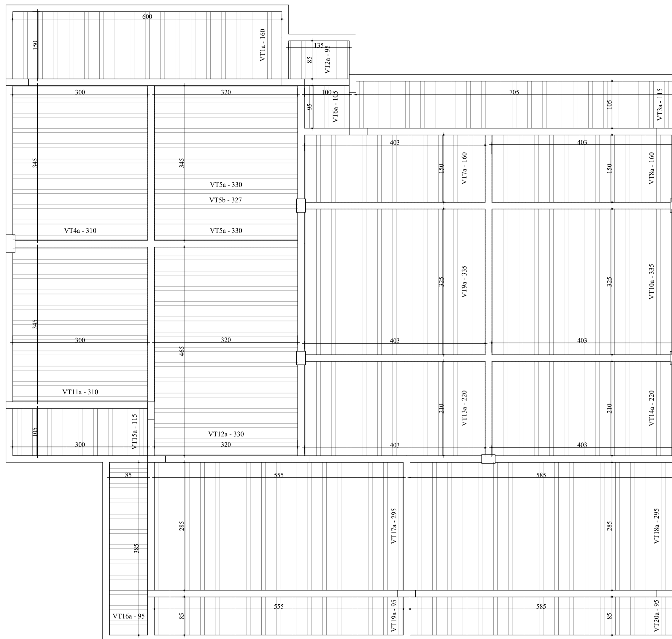
PLANTA DE VIGOTAS PRÉ-MOLDADAS Esc.: 1:50
