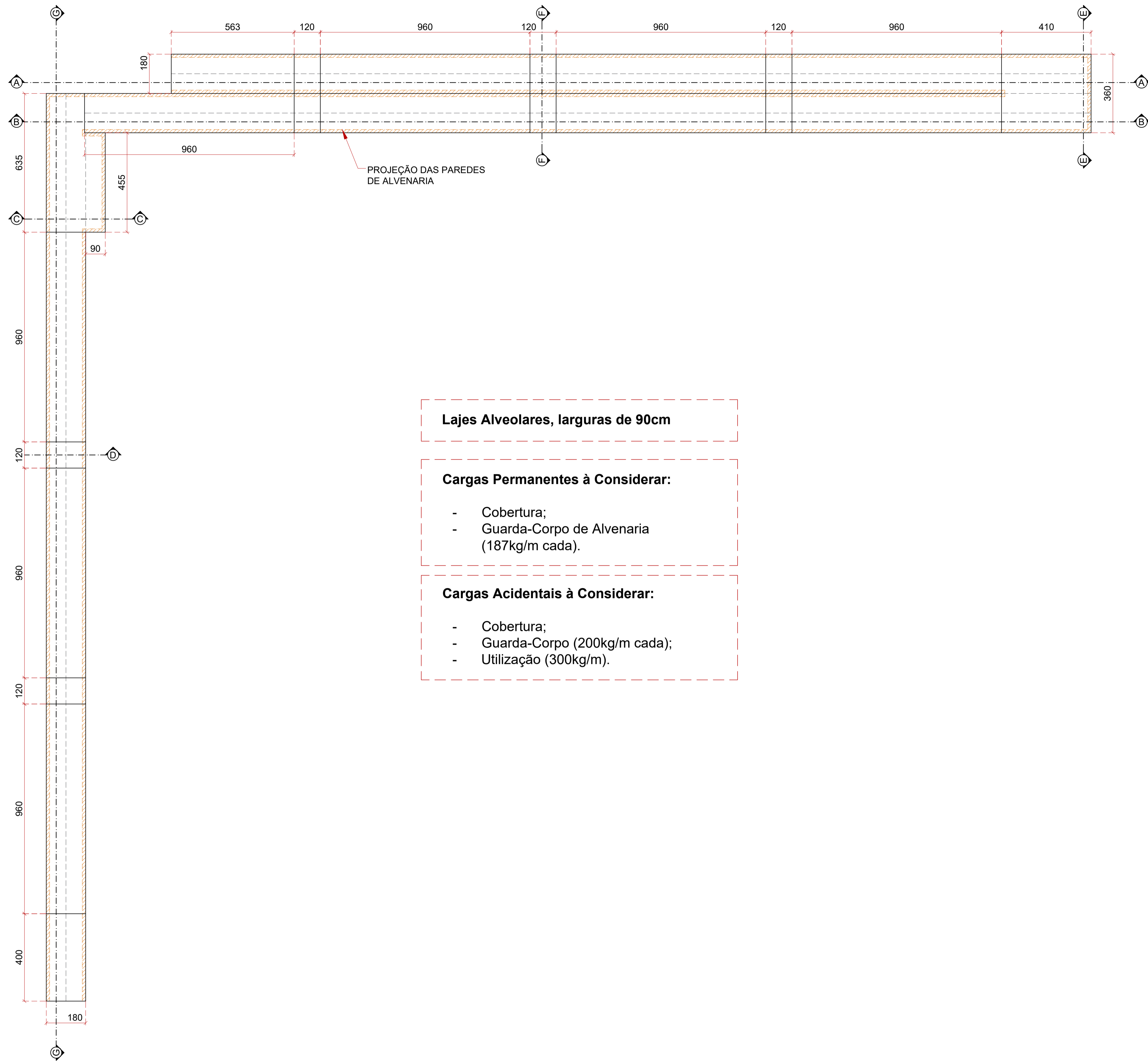
PLANTA LAJES ESC.: 1/100
