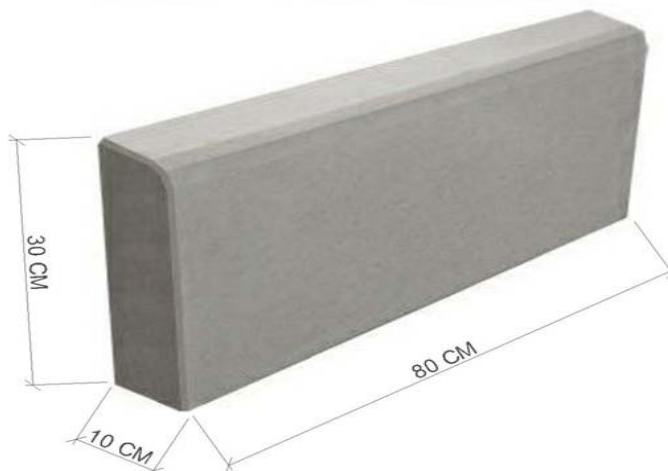
Figura 12 – Meio-fio arredondado
