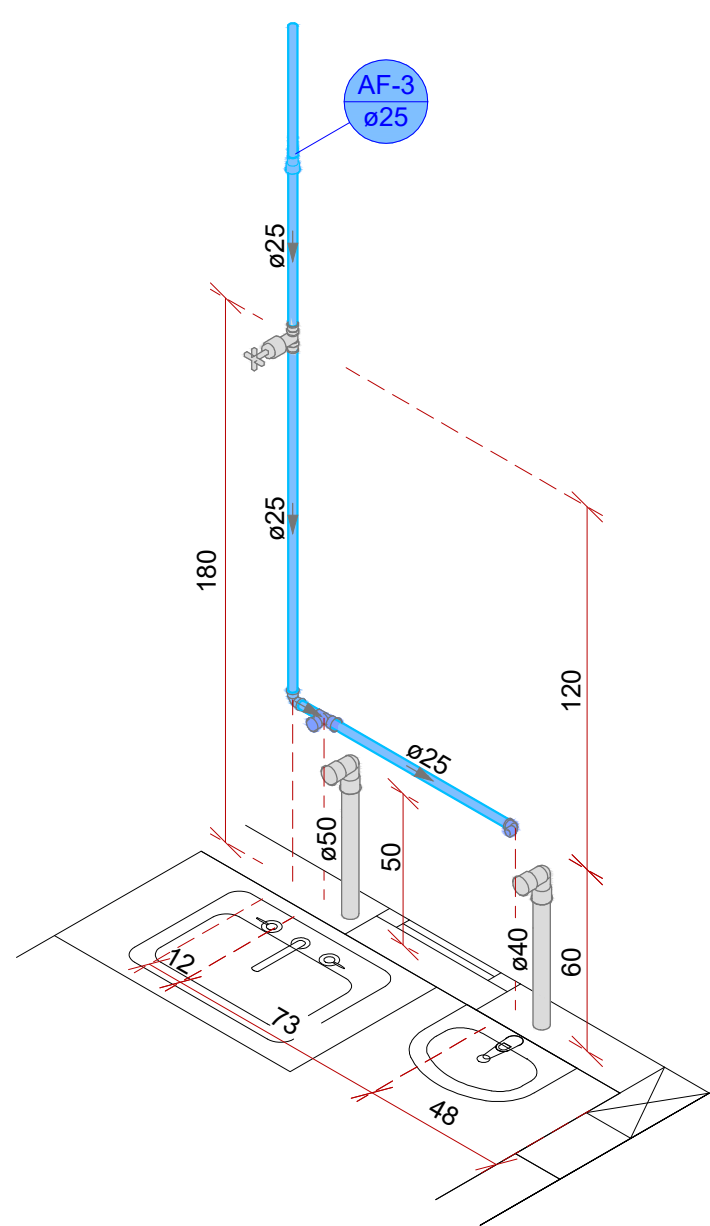
DETALHE H1 ESC.: 1/25
