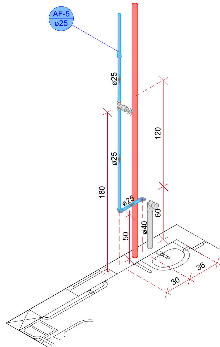
DETALHE H6 ESC.: 1/25
