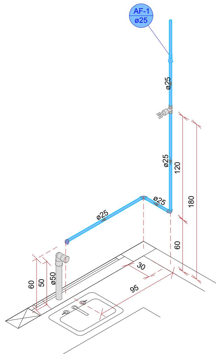
DETALHE H2 ESC.: 1/25
