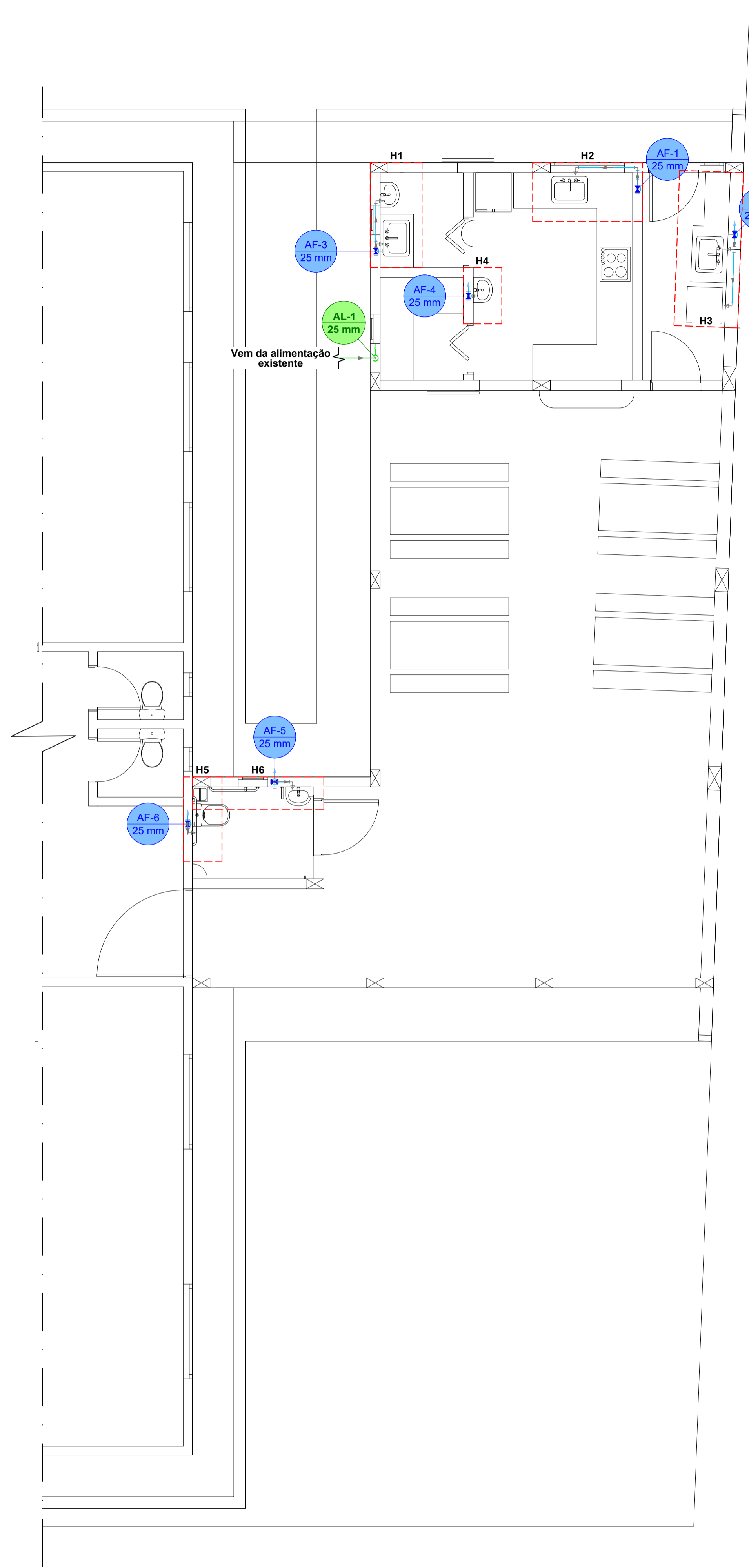
PROJETO HIDRÁULICO - PAV. TÉRREO ESC.: 1/50
