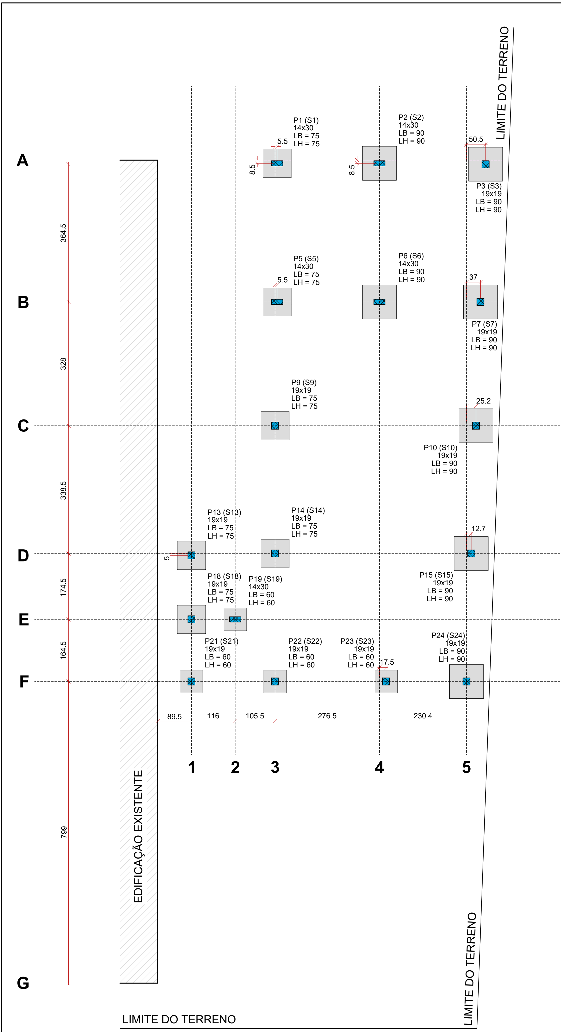
PLANTA DE LOCAÇÃO ESC.: 1:50
